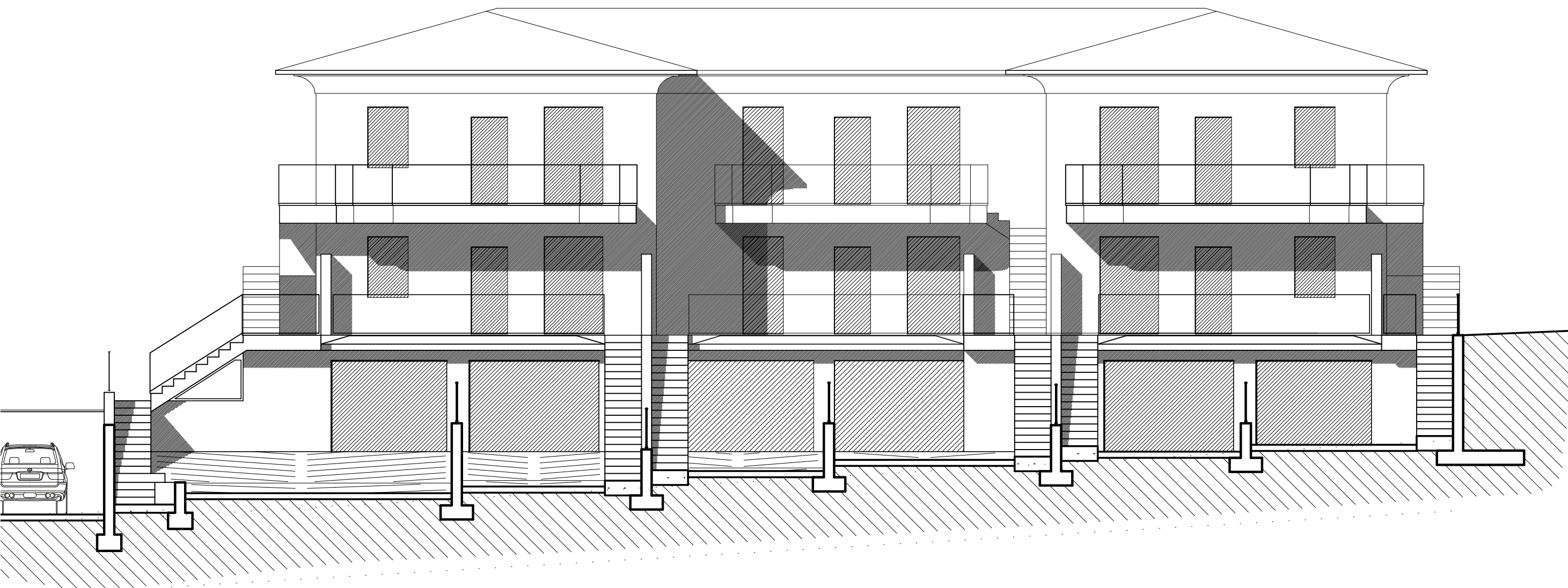
PROSPETTO FRONTALE scala 1:100
