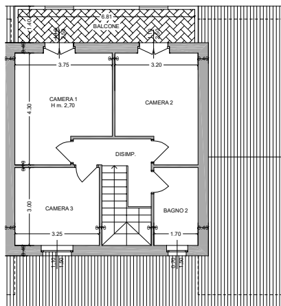
PIANO PRIMO
